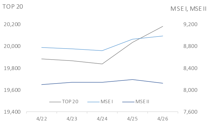
MSE Индекс
